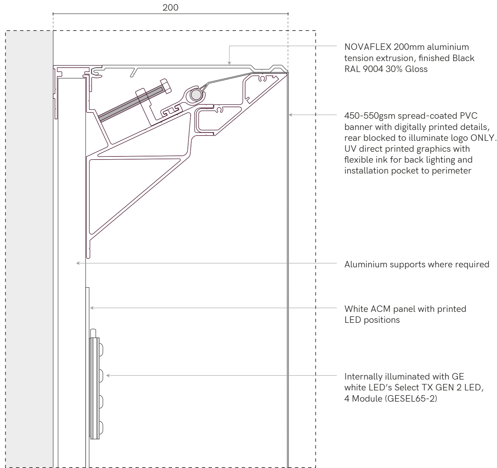
SECTION | 1:2
