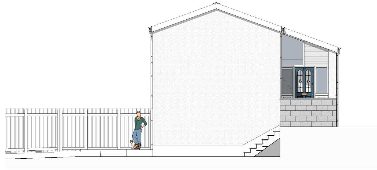
E 1 :: EXISTING SIDE ELEVATION scale: 1:100
