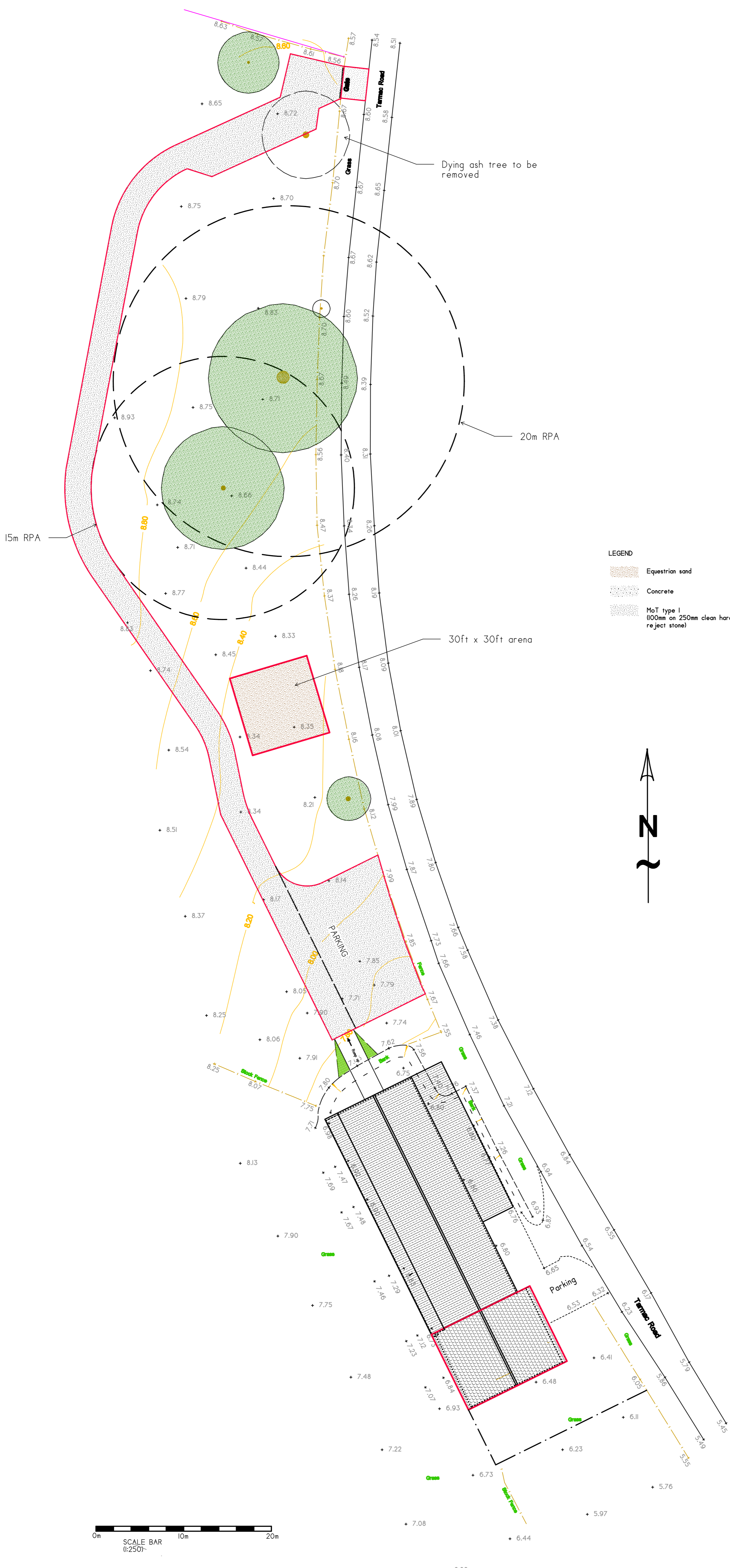
Site Plan 1:250
