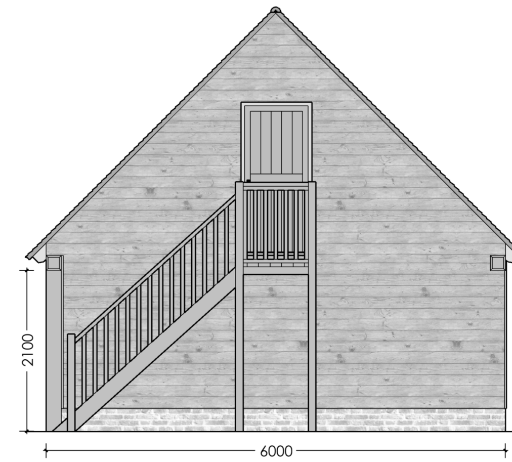
Right Elevation
