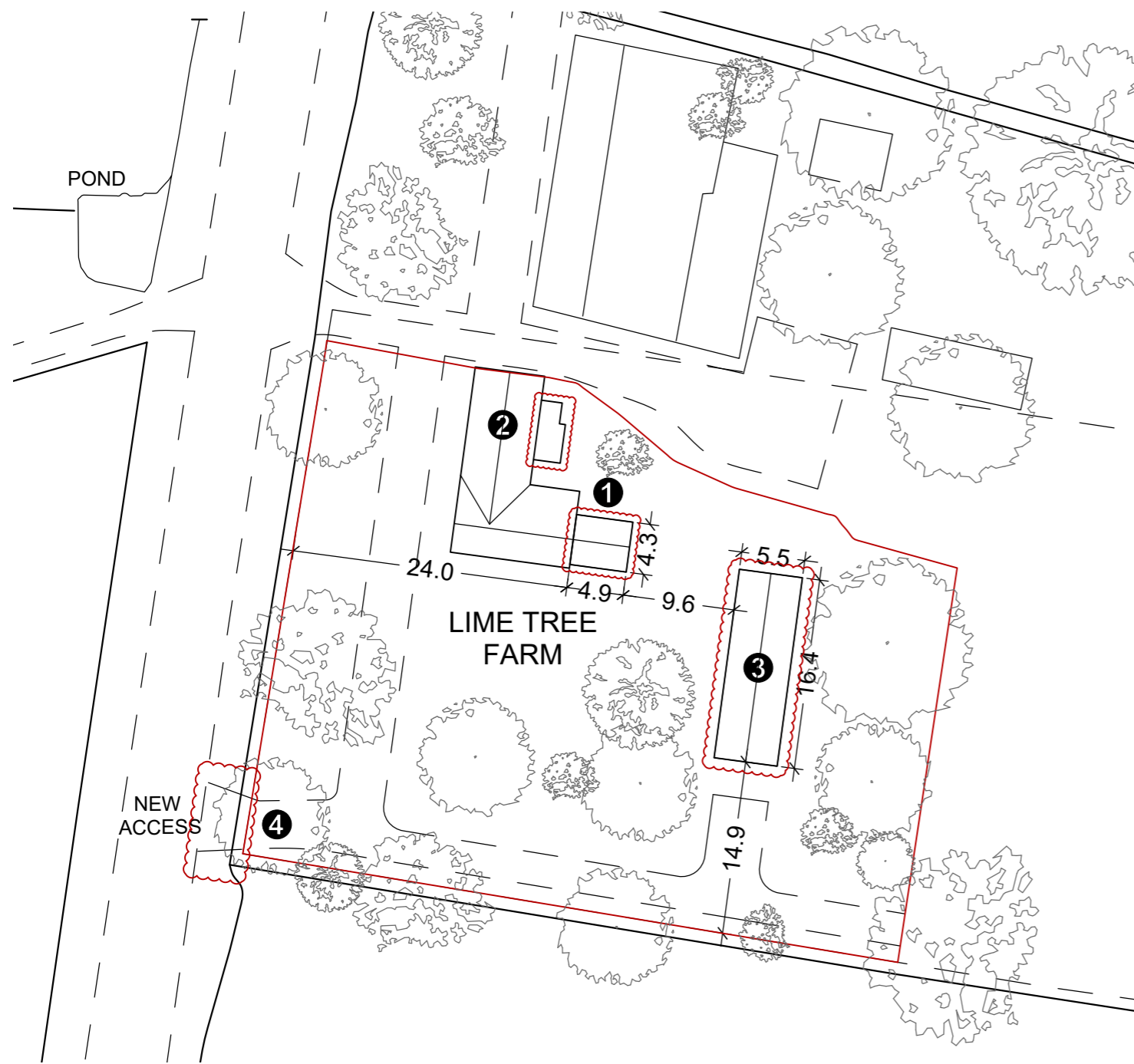
SITE PLAN 1:500
