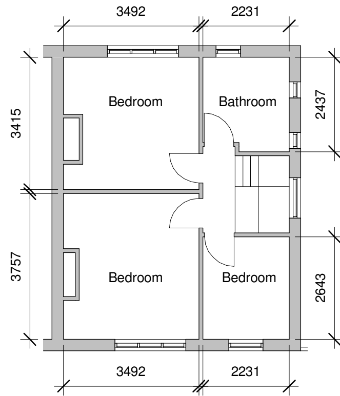
First 1 : 100
