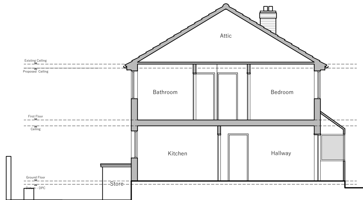
Existing - Section A1
