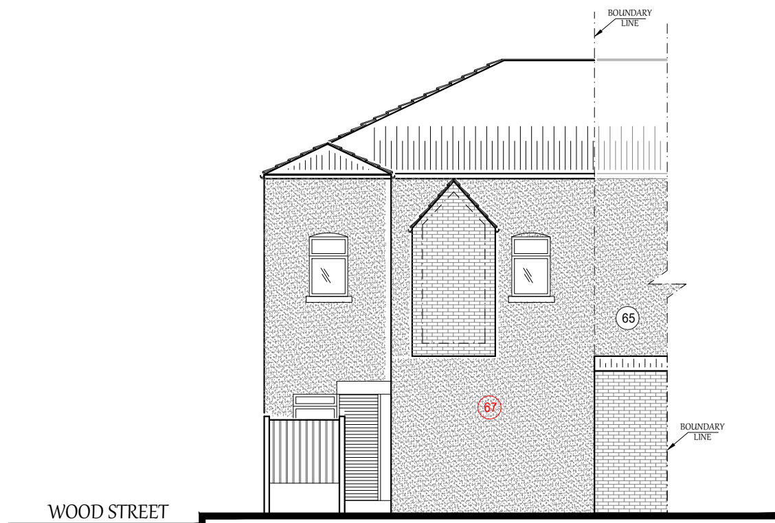
EXISTING VIEW 1 SCALE: 1/100 @A3
