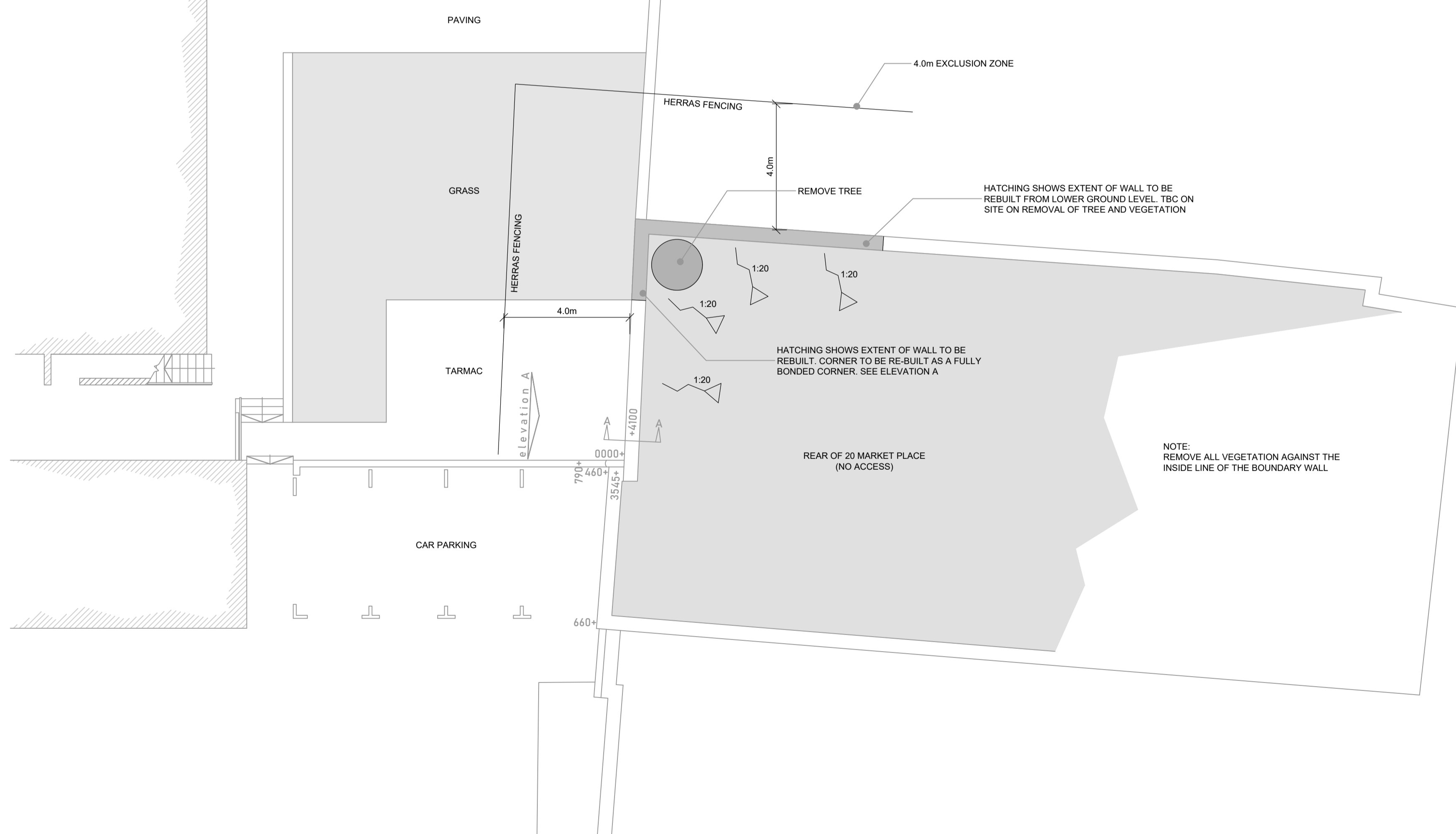
PLAN 1:100
