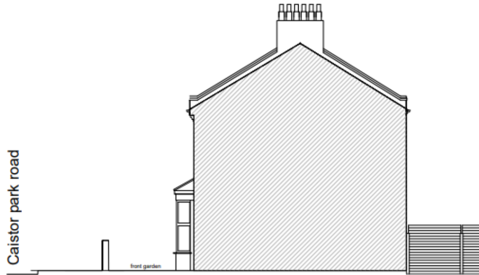
Existing Flank Elevation
