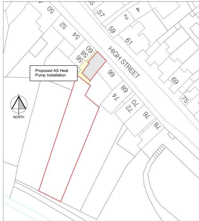
Site Plan 1:500
