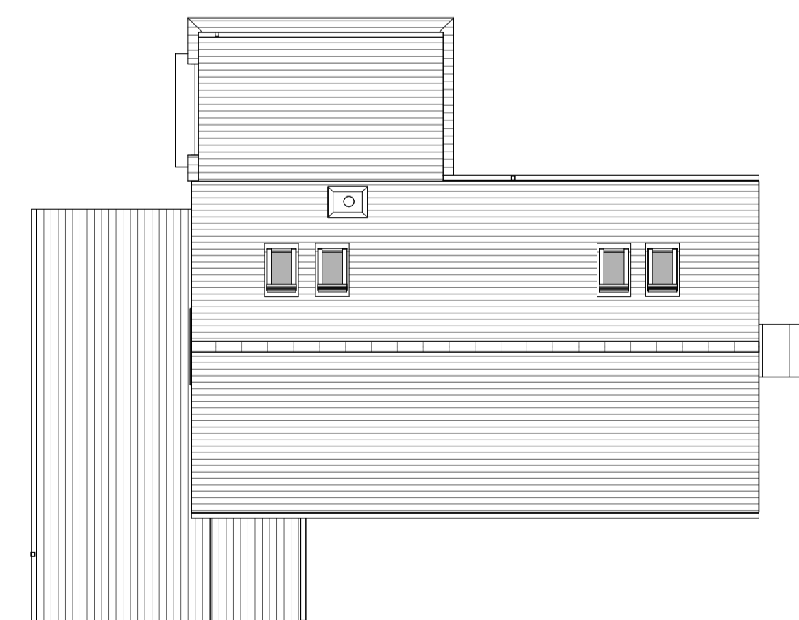
7 Roof Plan 1 : 100
