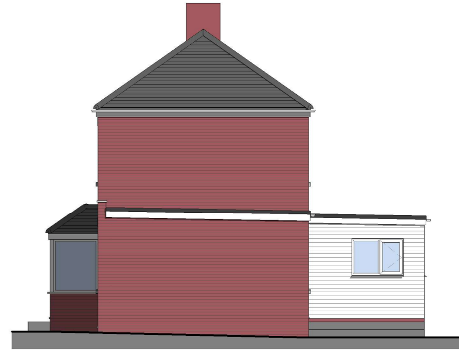
2 RHS Elevation 1 : 100
