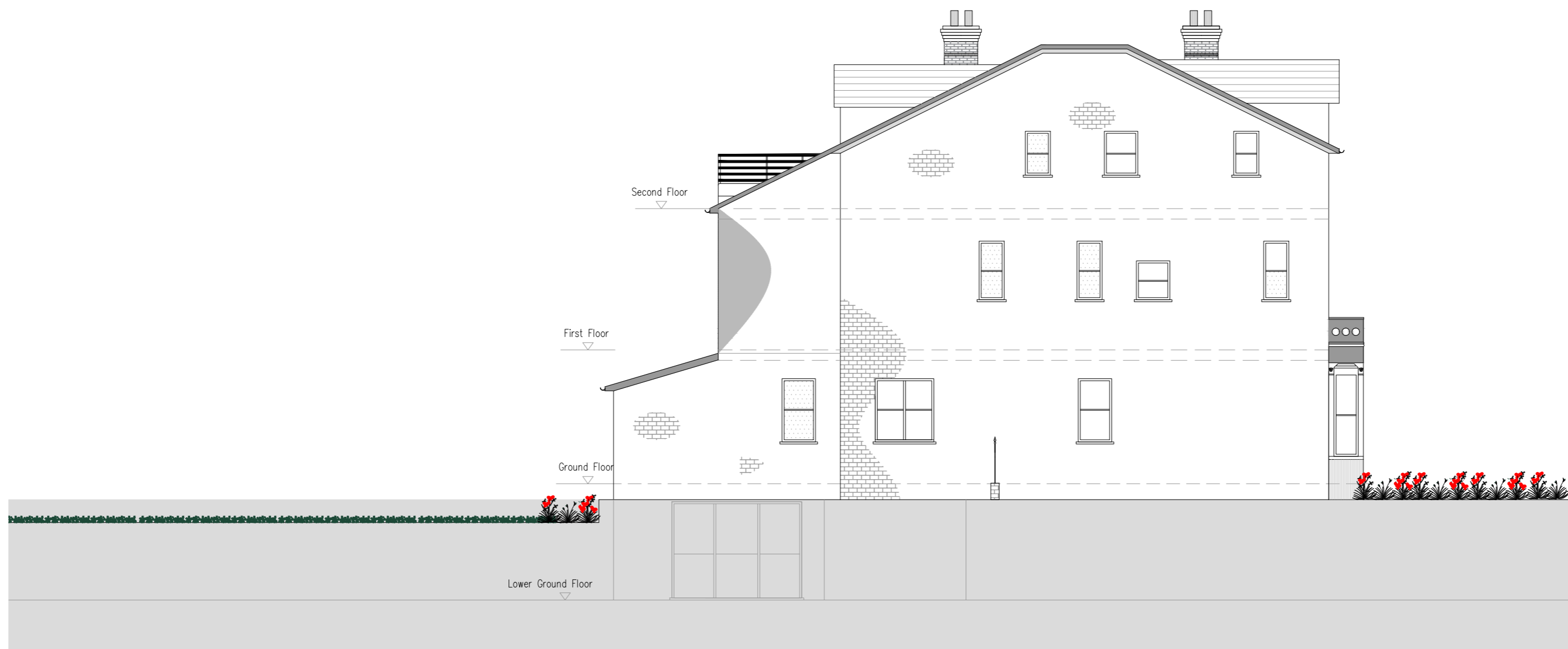
EXISTING SIDE ELEVATION - B Scale: 1:100
