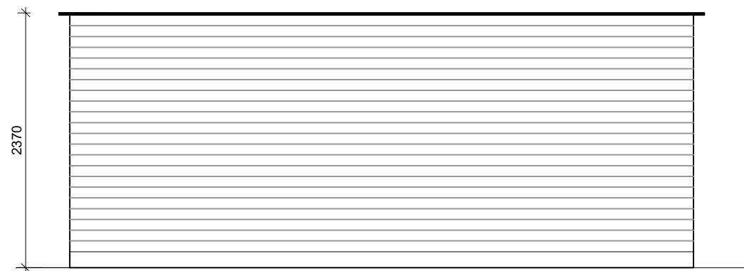
ELEVATION A-B
