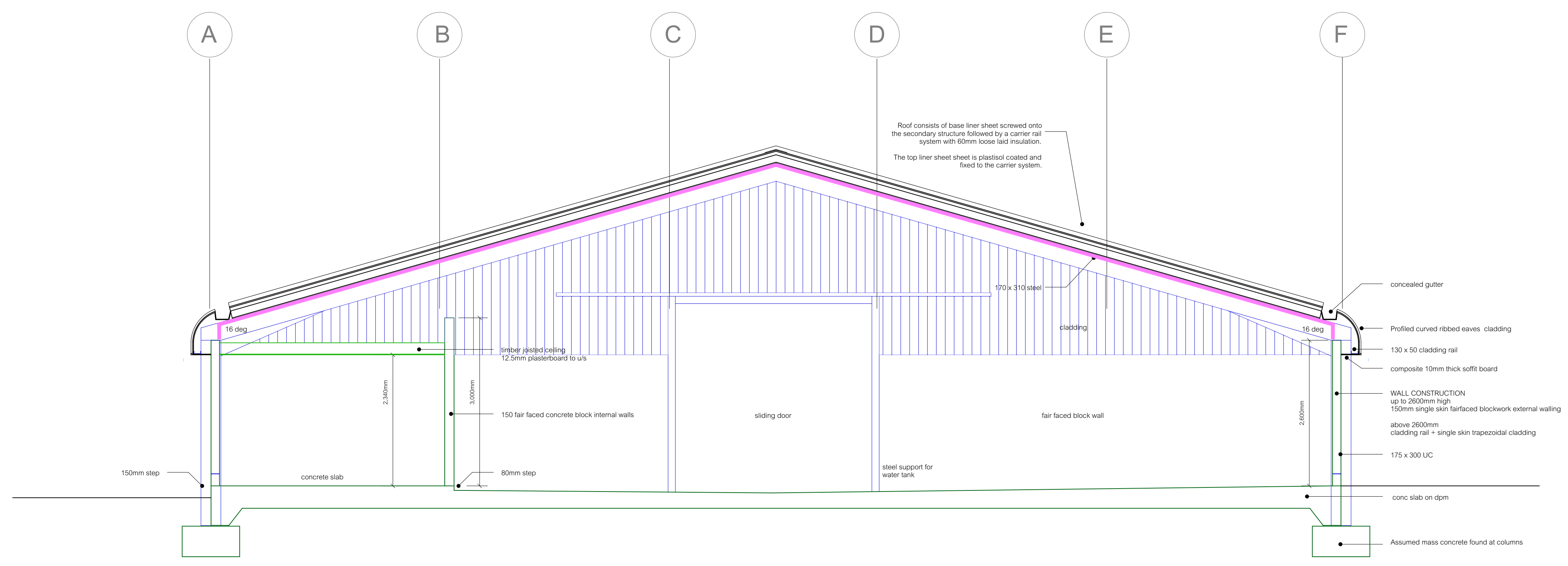
SECTION A-A
