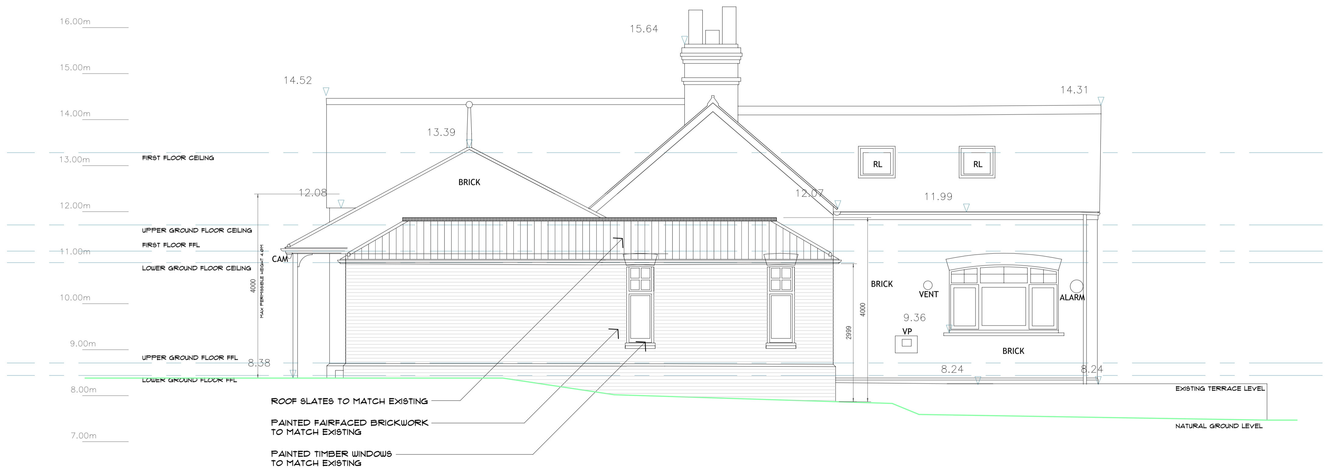
RIGHT FLANK ELEVATION
