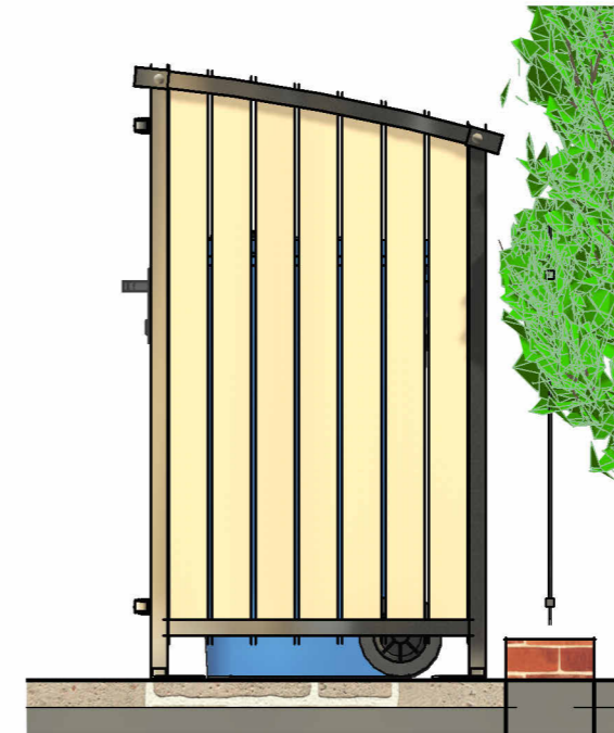
5 LEFT Scale 1:20
