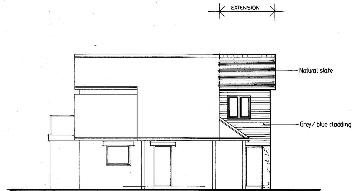
SE elevation 1:100
