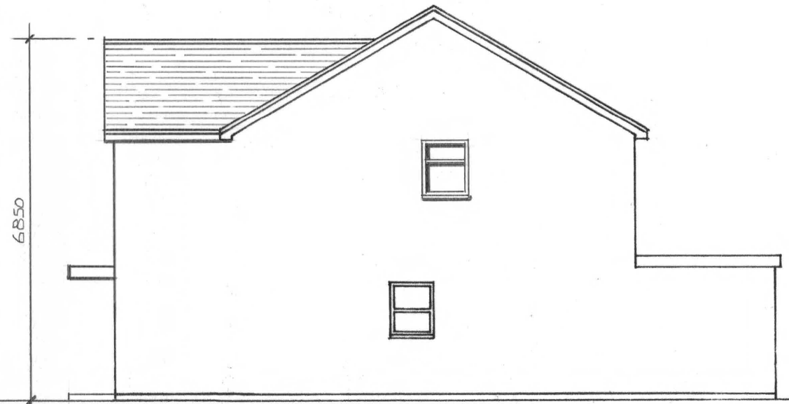
RIGHT ELEVATION
