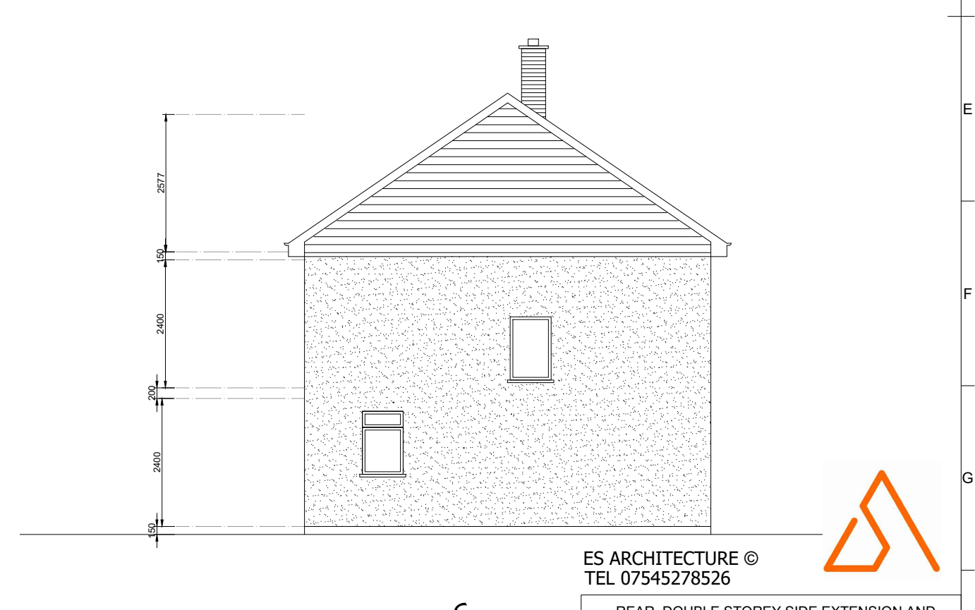
4 SIDE ELEVATION - EXISTING Scale: 1:100
