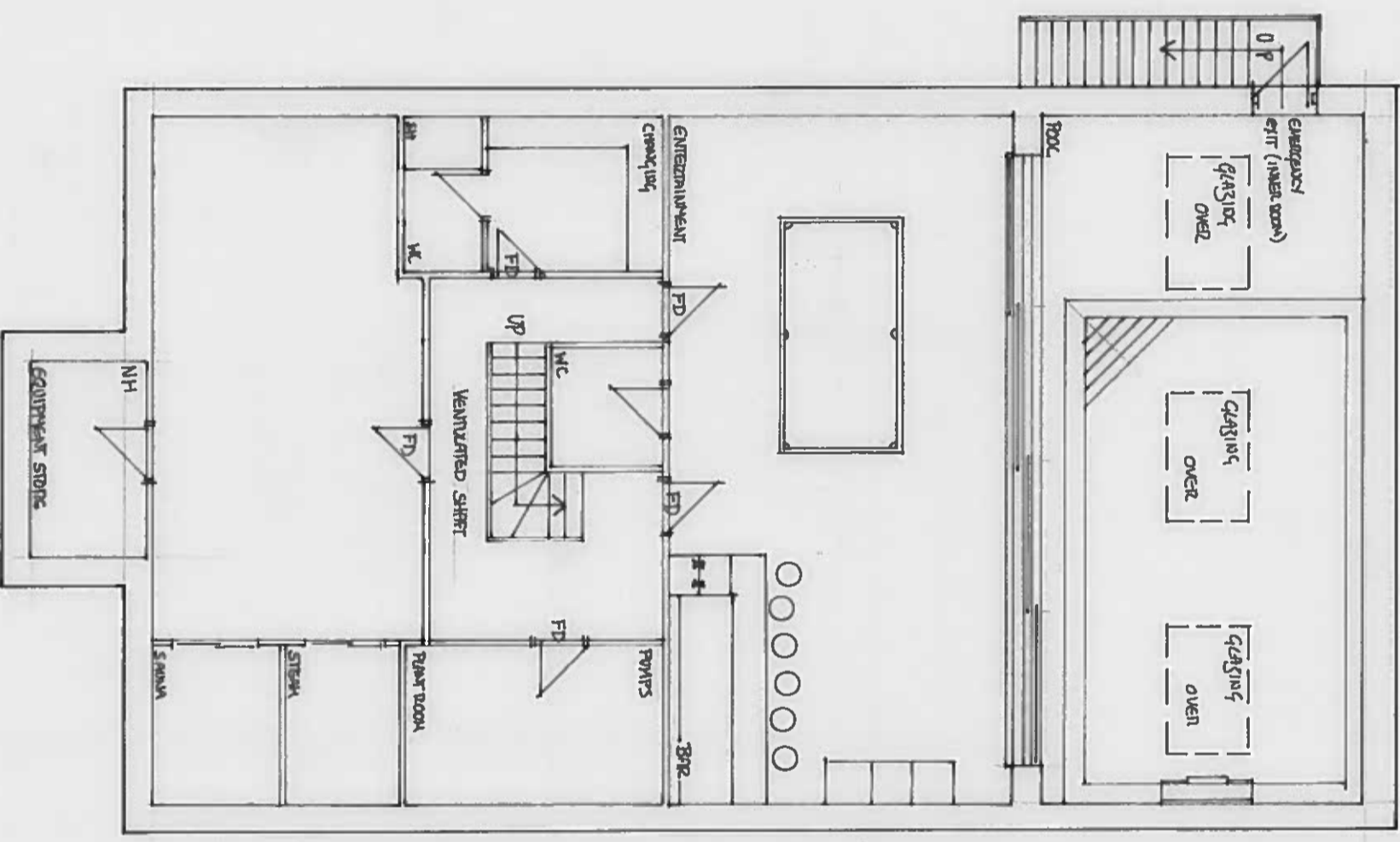
BASEMENT PLAN 1:100 GA3
