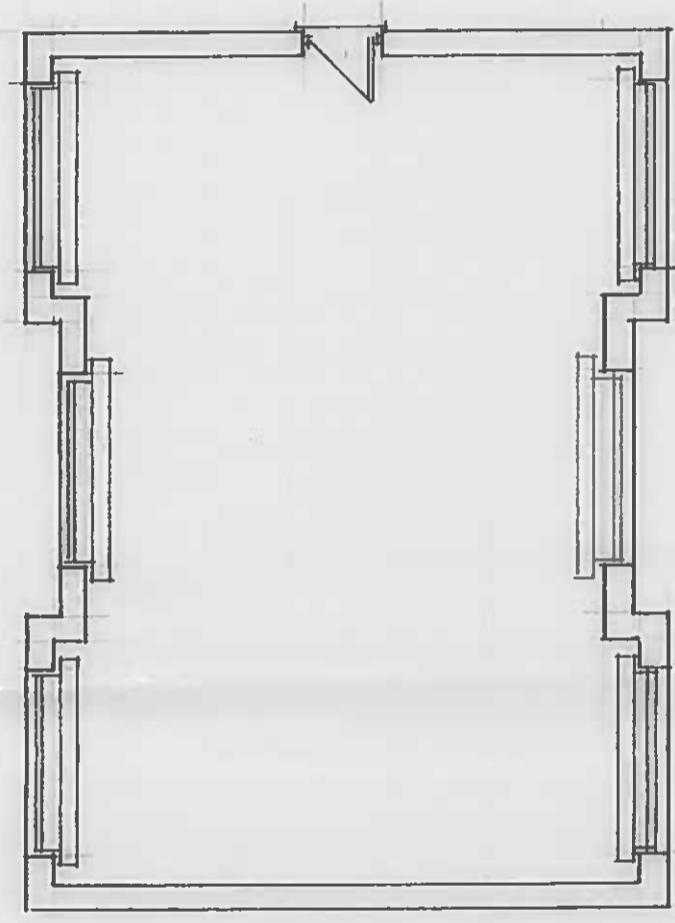
PLAN 1:100
