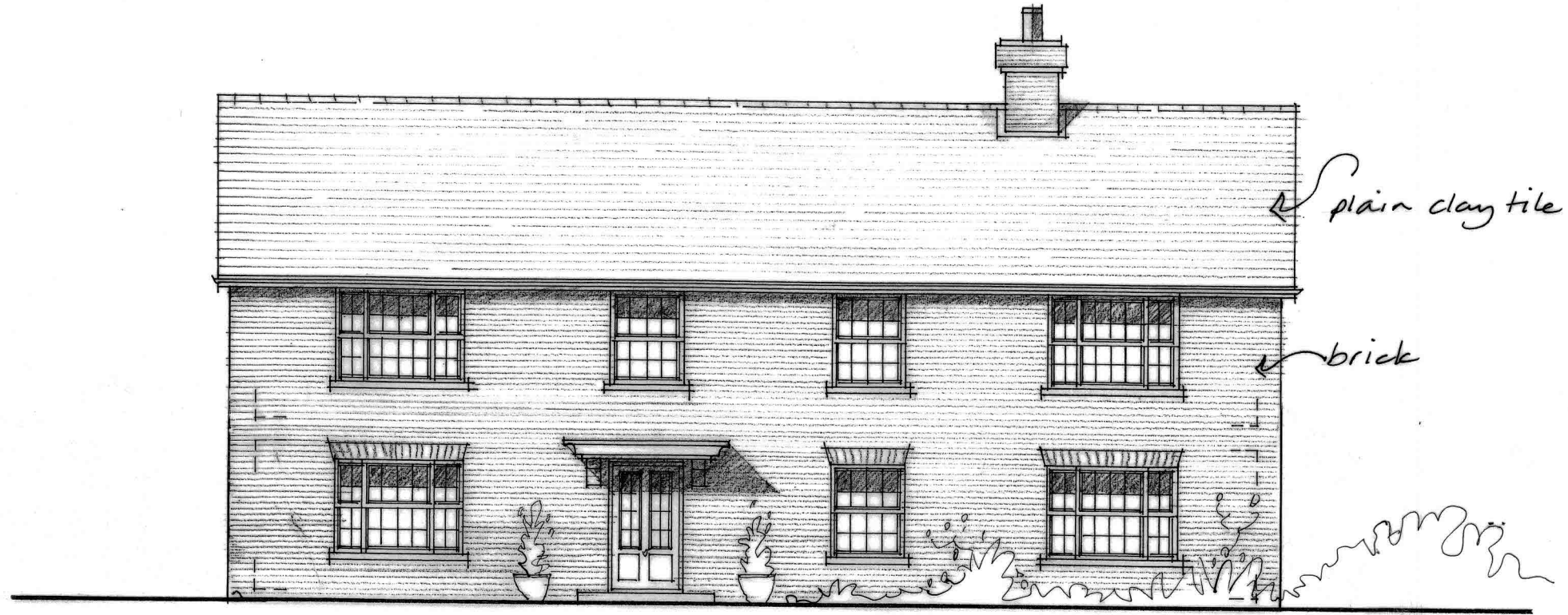
N O R T H W E S T E L E V A T I O N
