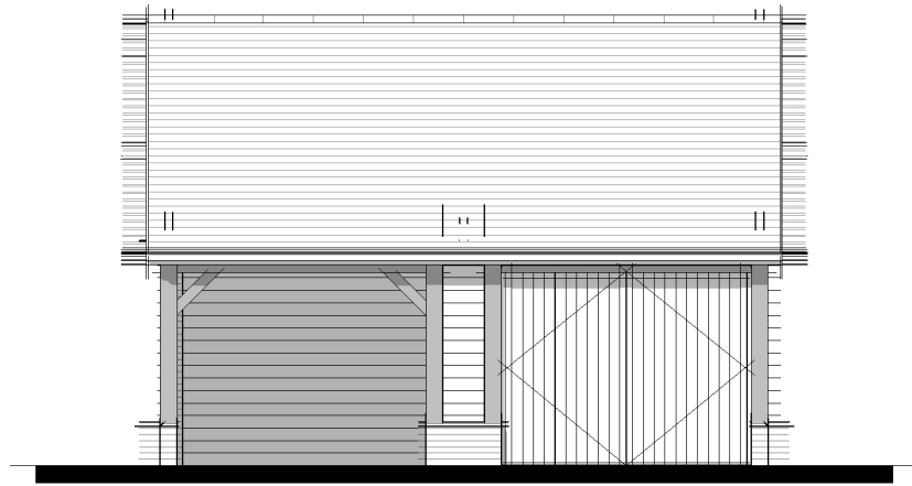
Front 1 : 100
