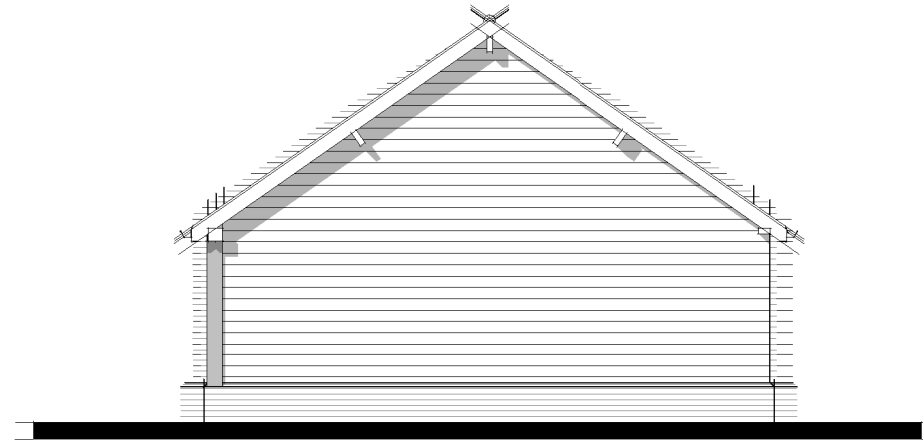
Side 1 1 : 100
