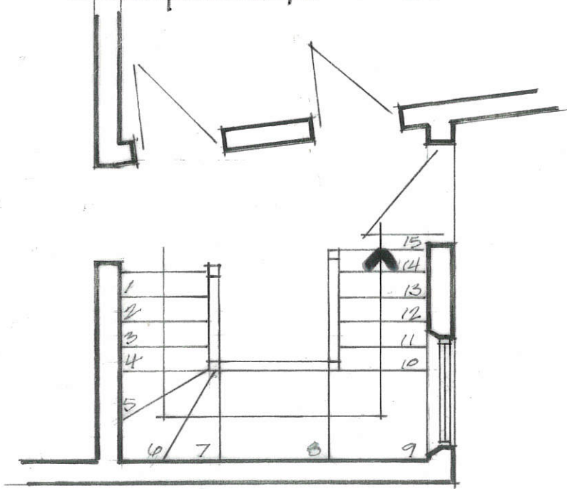
RF PLAN 1:50
