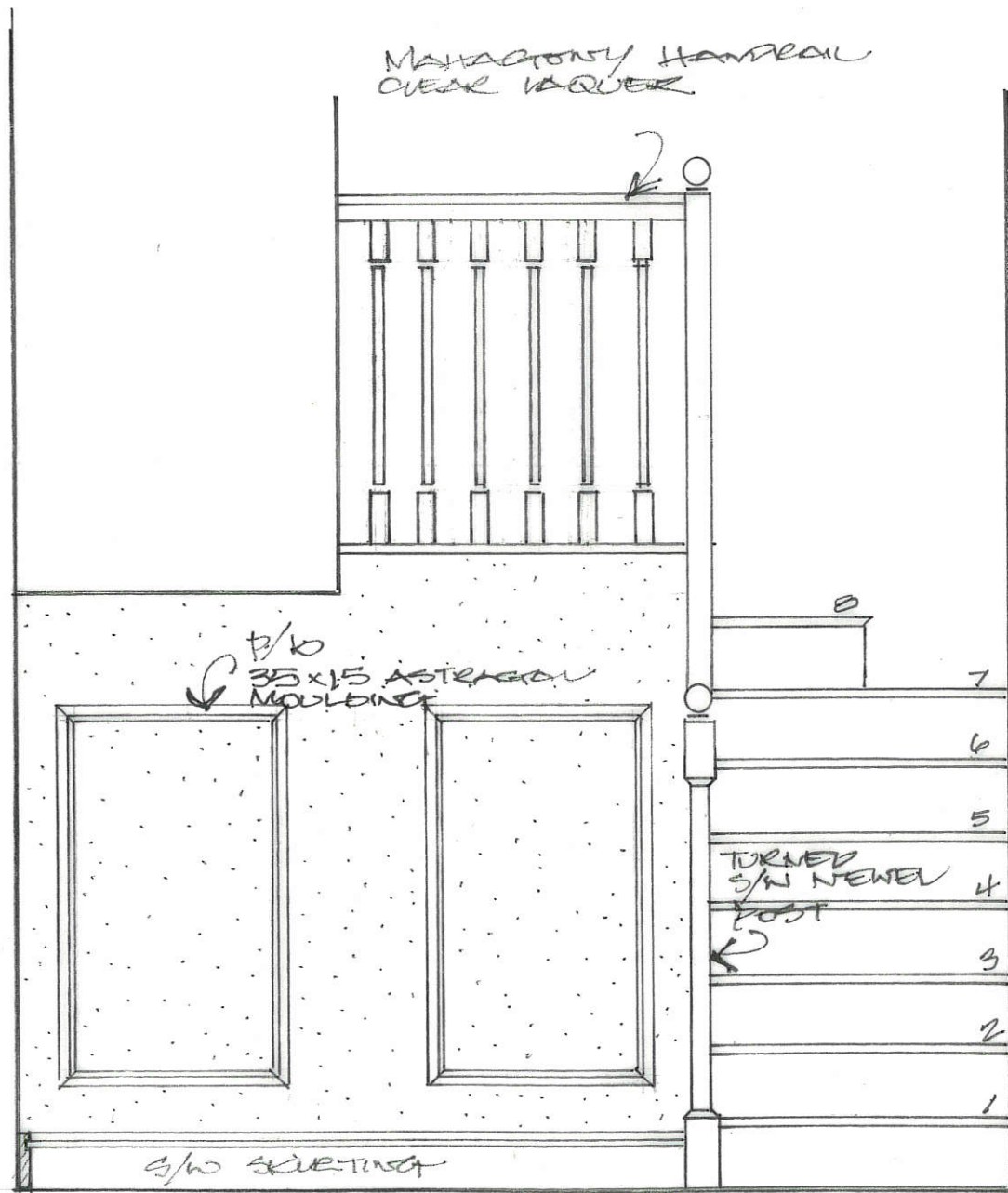
ELEVATION A-A
