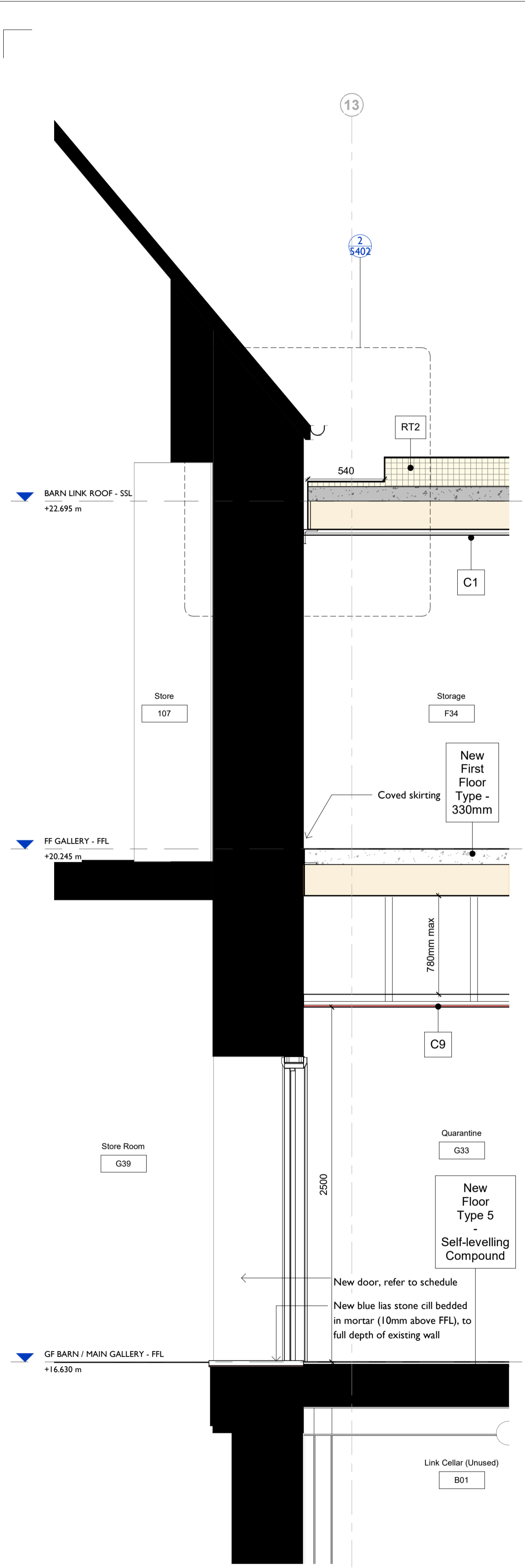
Ladder Section 5 - Section DD 1 : 20
