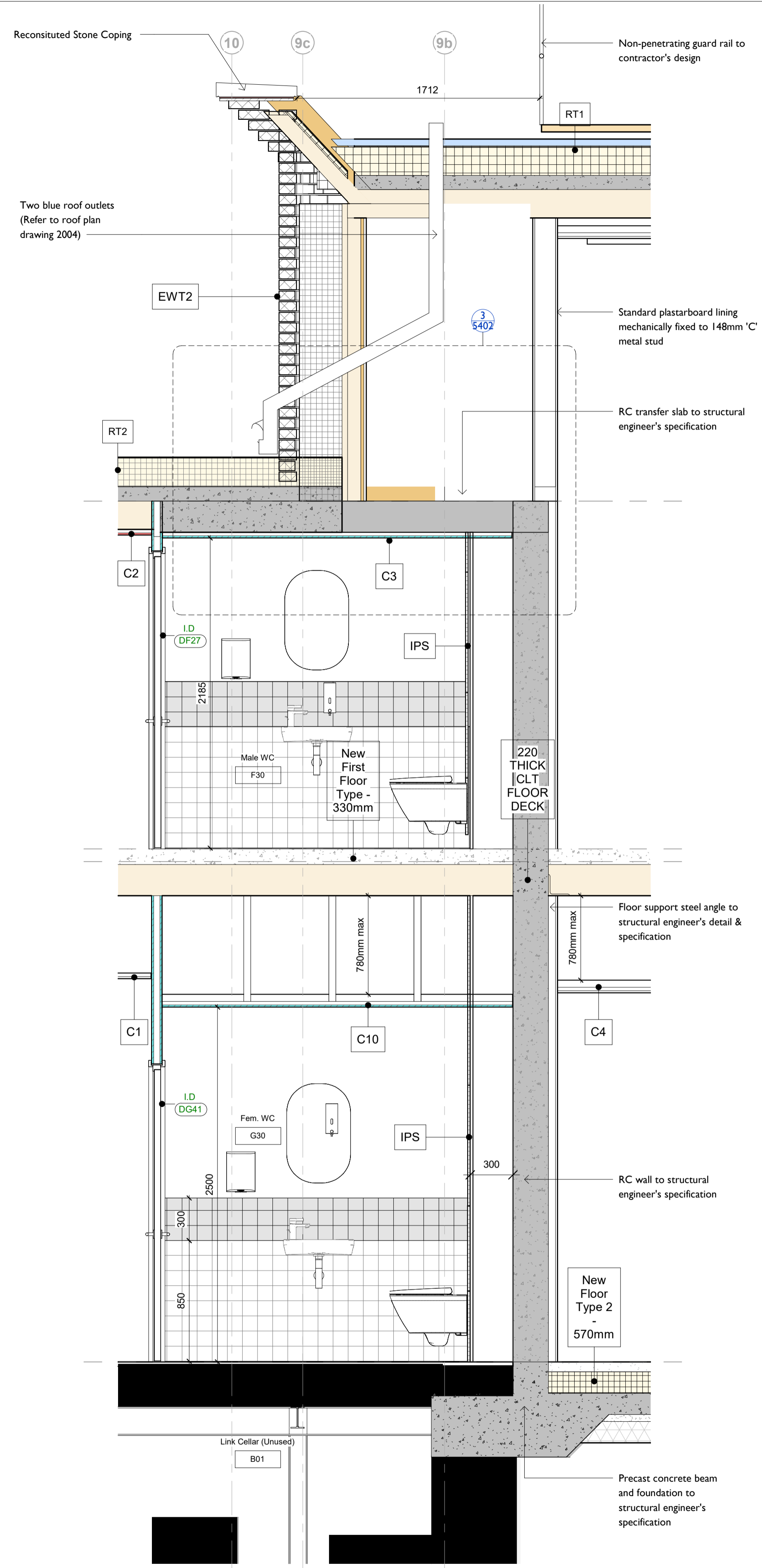
Ladder Section 6 - Section DD 1 : 20
