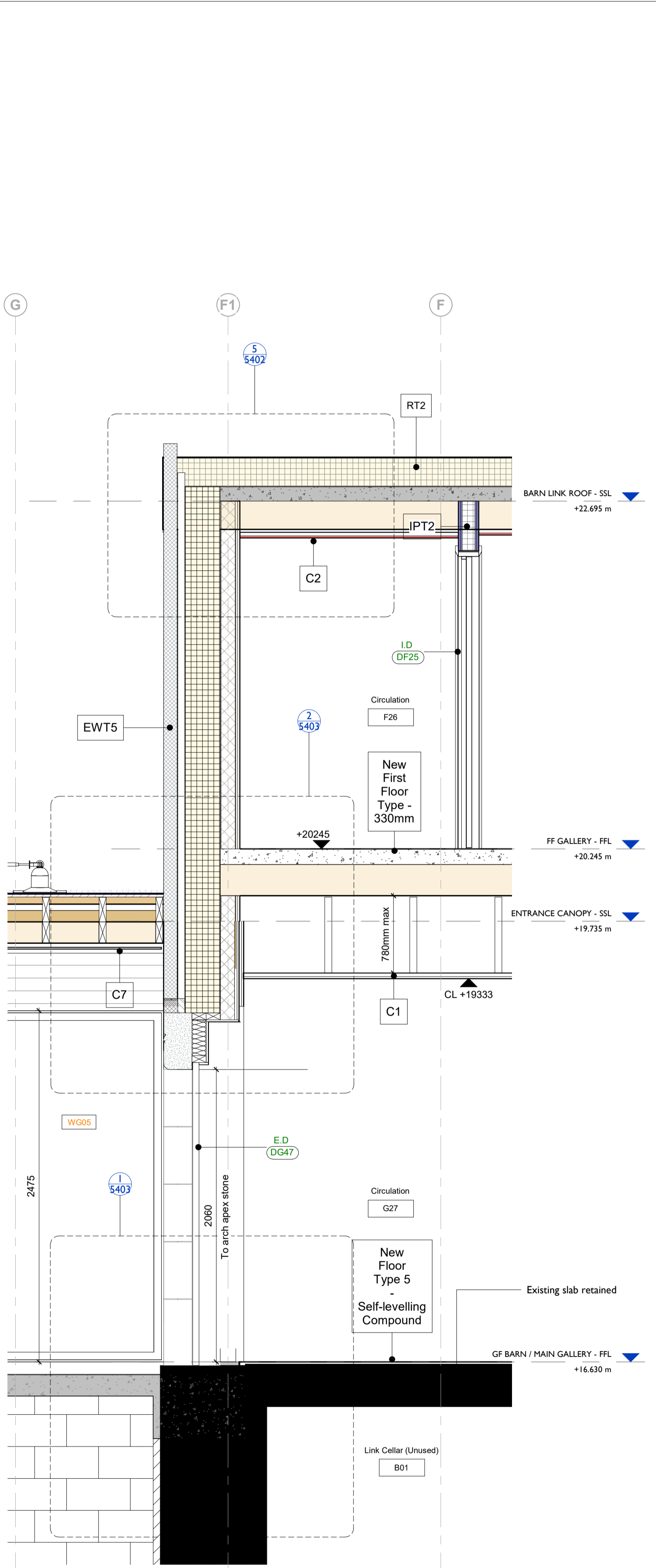
Ladder Section 7 - Section FF 1 : 20
