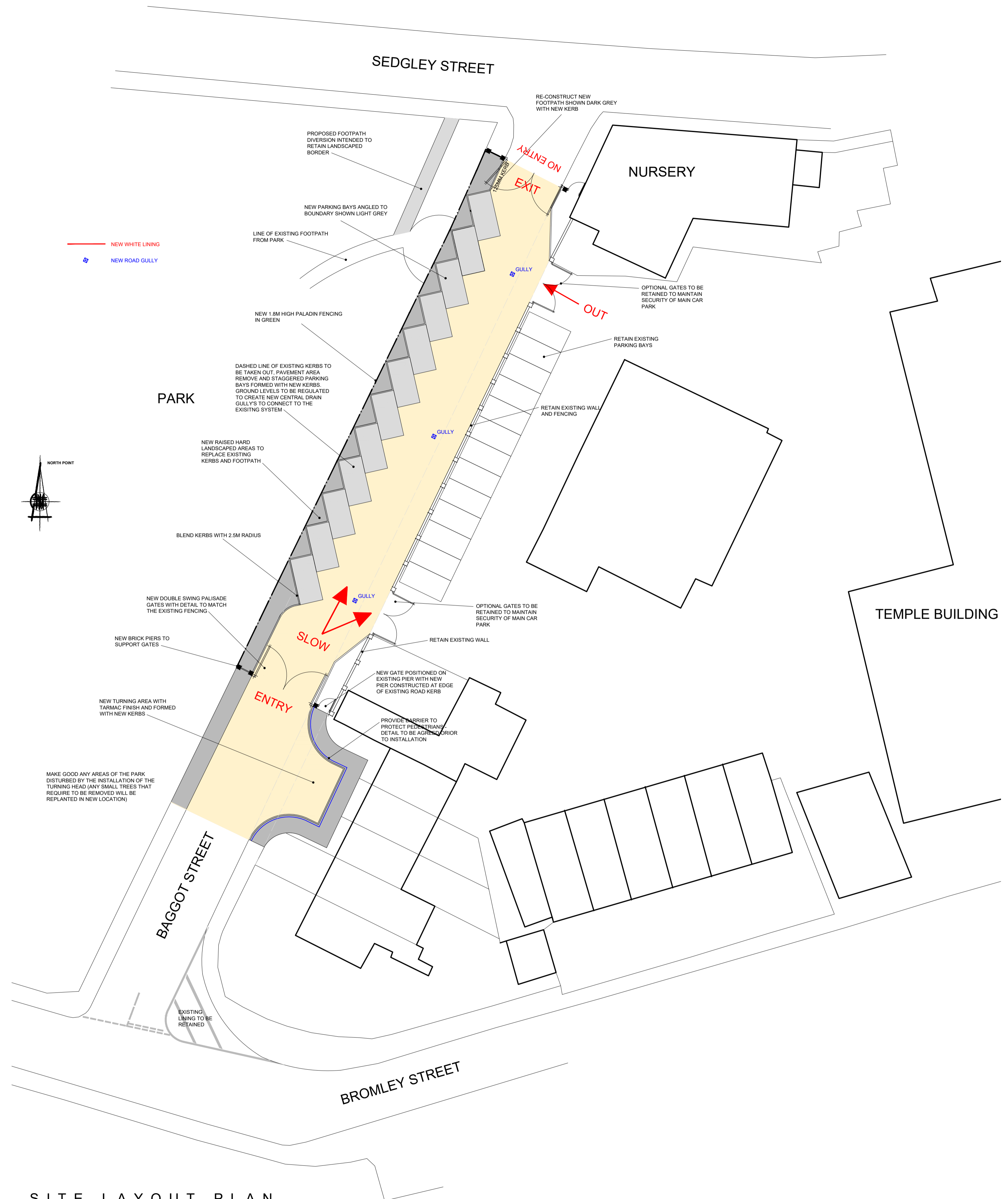
SITE LAYOUT PLAN 1:250@A1
