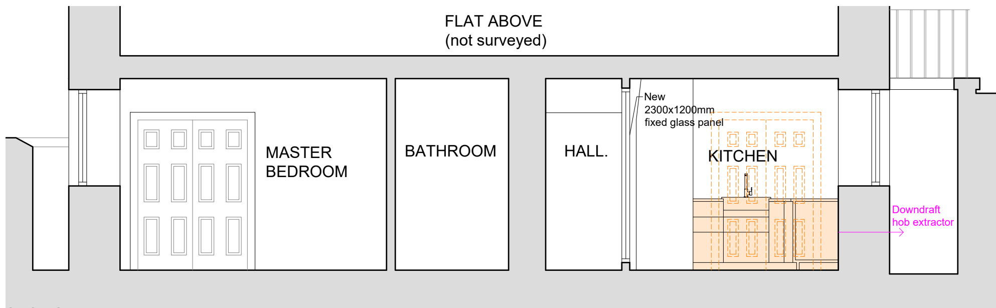
SECTION A-A
