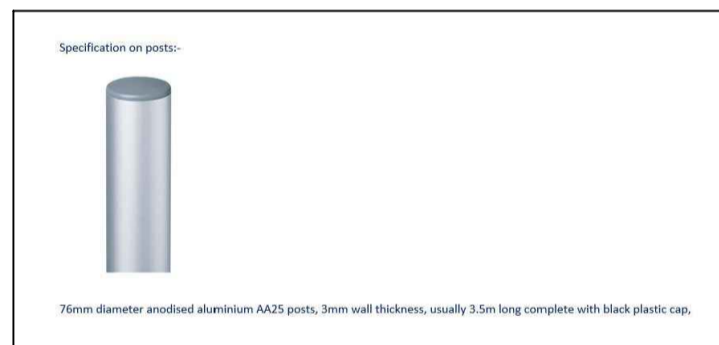
New Post Specification N.T.S
