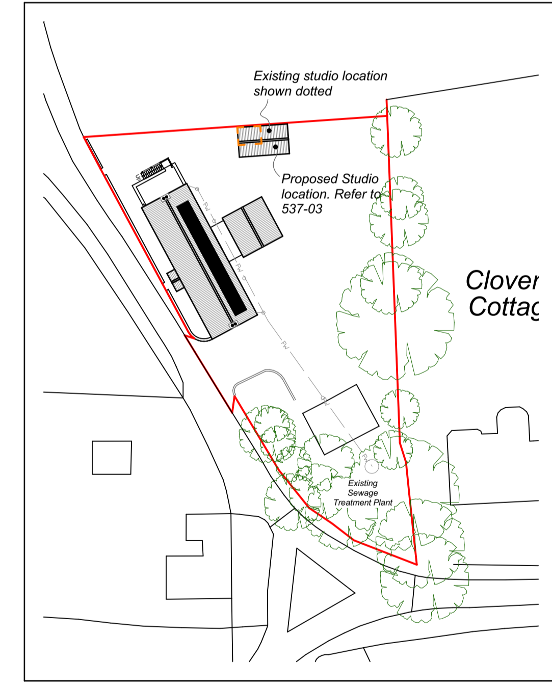
CHA Site Plan 1:500
