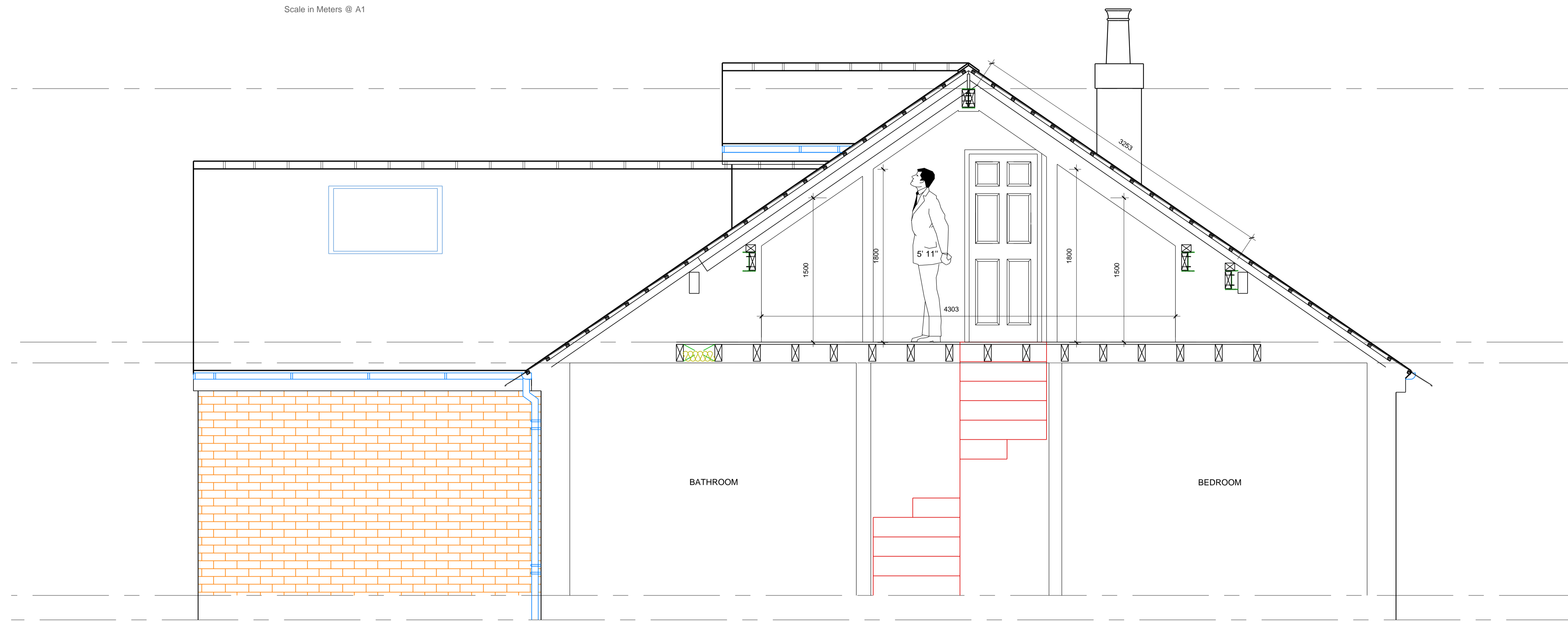
(A-A) Section A-A Scale: 1:25 @ A1
