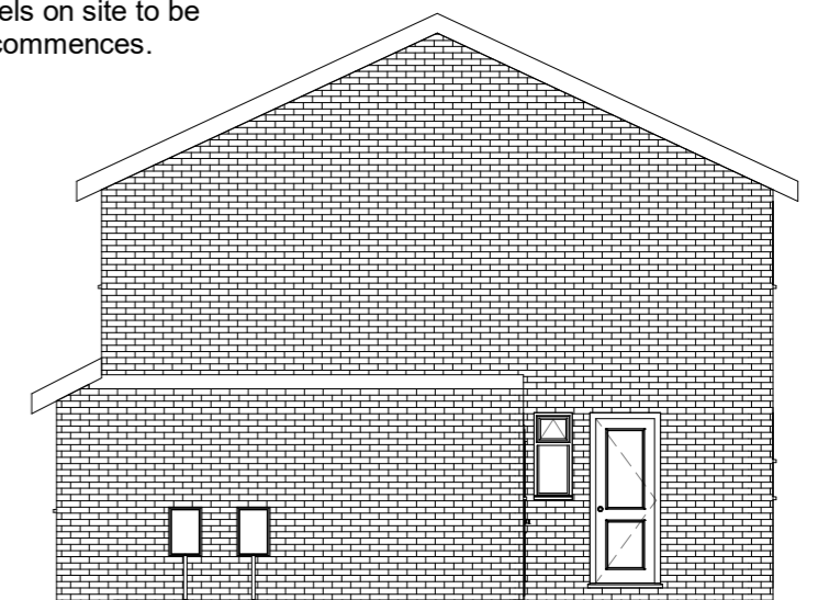
3 Garage Gable 1 : 100
