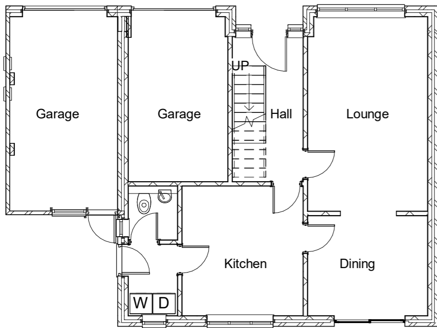
1 dpc 1 : 100
