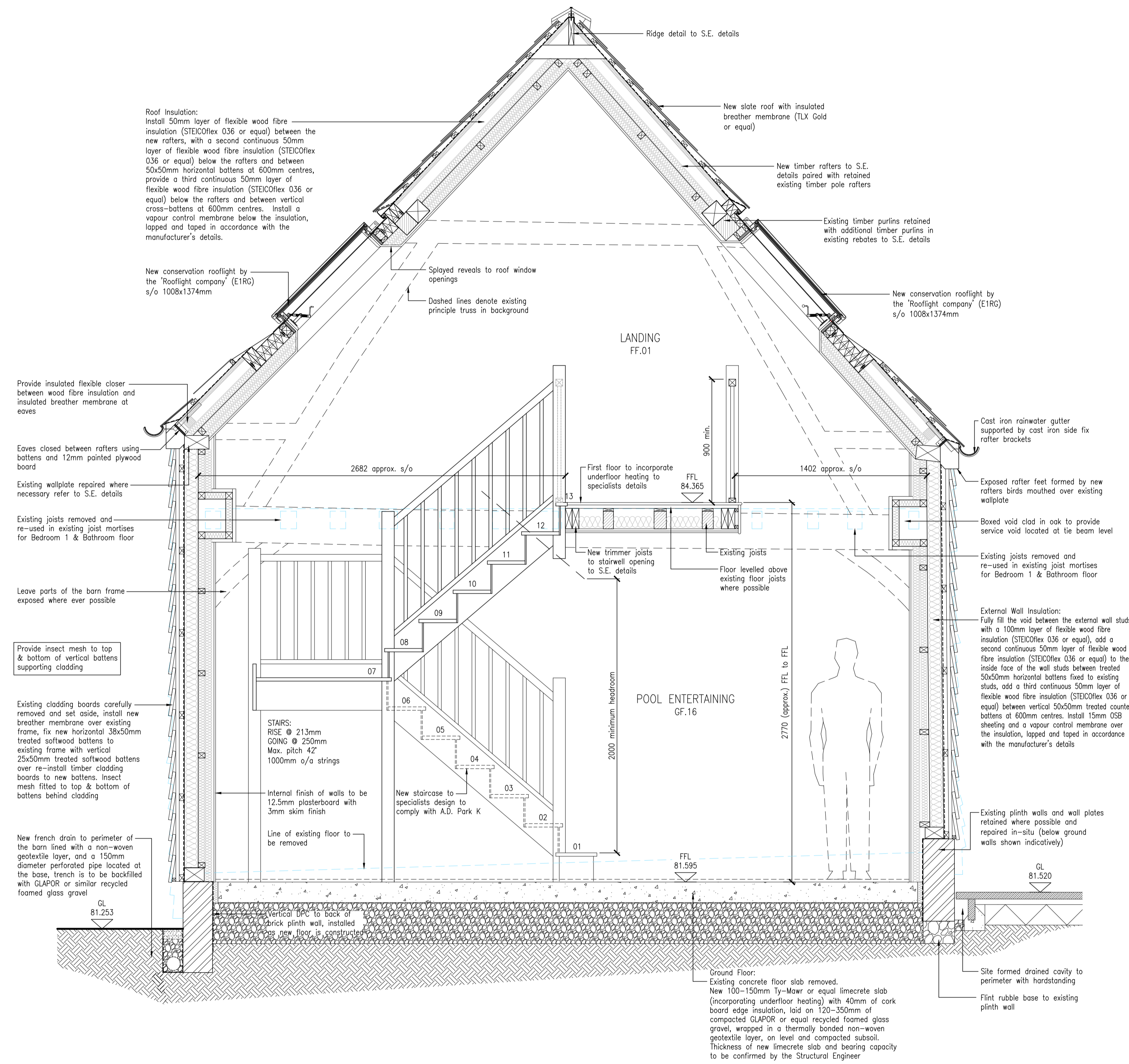
SECTION G-G BARN
