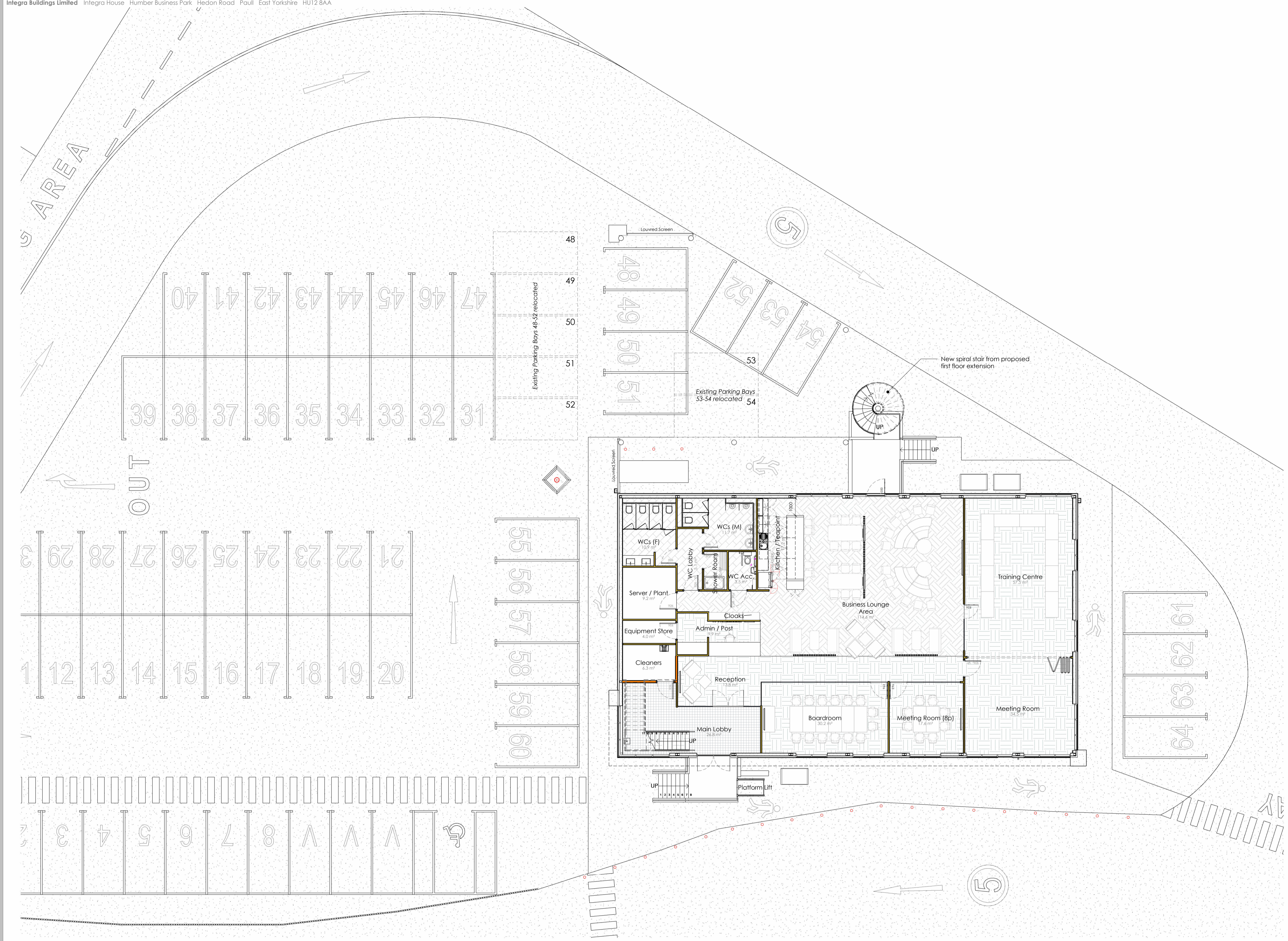
Site Plan - Extension 1 : 100
