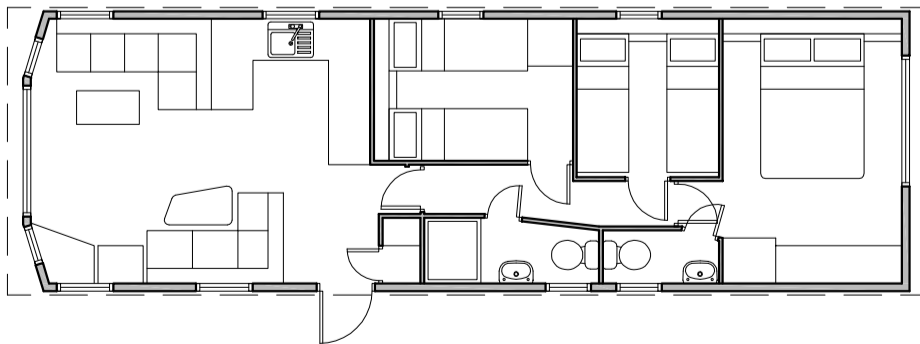
CYNLLUN LLAWR DDAEAR GROUND FLOOR PLAN
