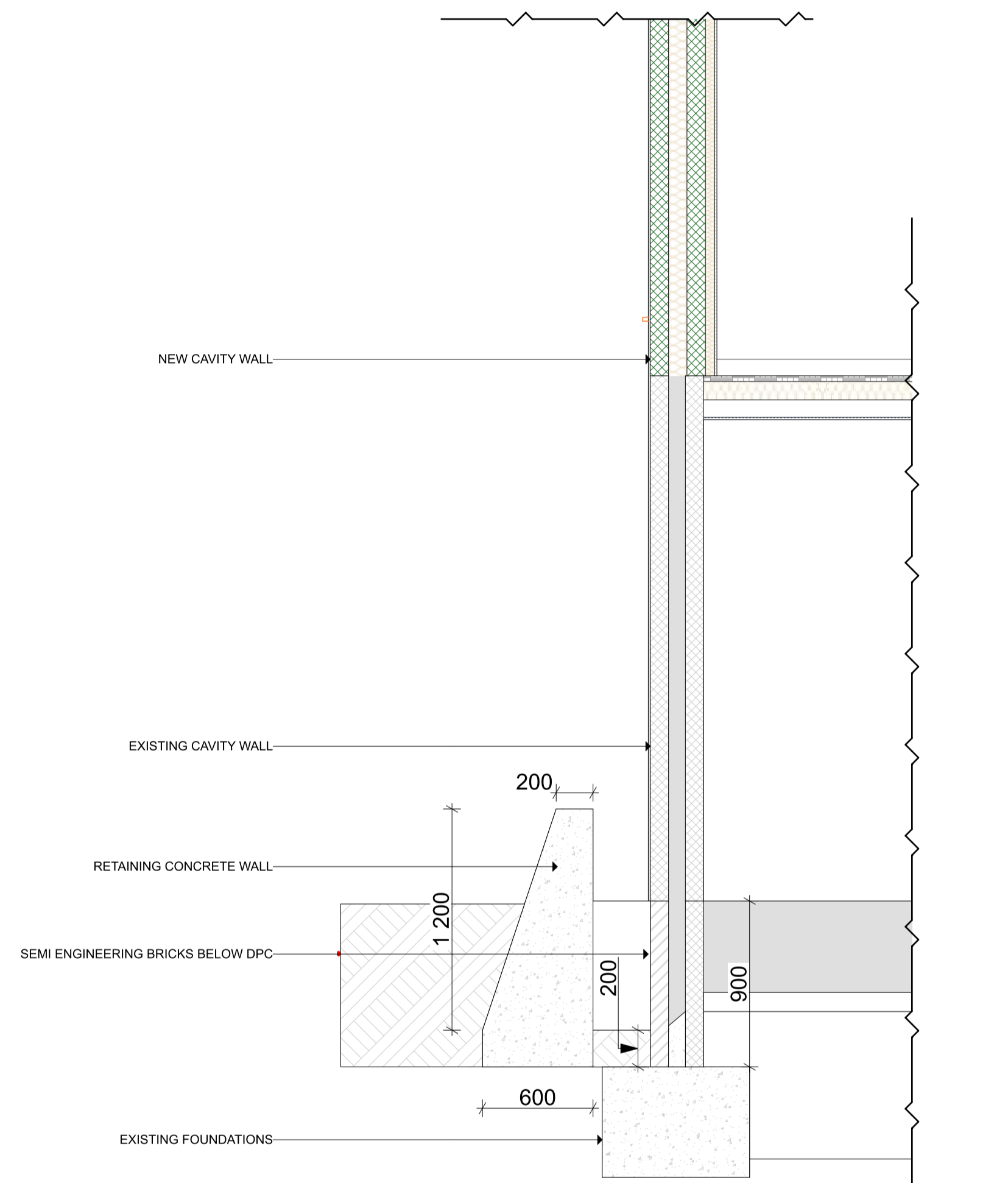
SECTION A-A
