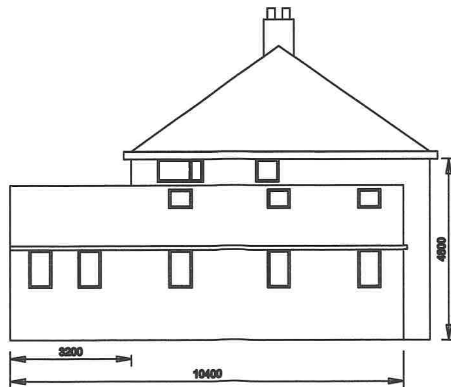
S. W. Facing elevation
