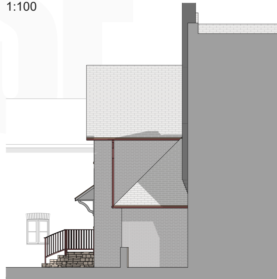
E3 Side Elevation 1:100
