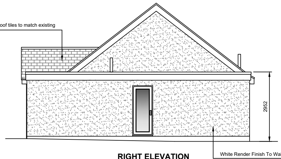
RIGHT ELEVATION
