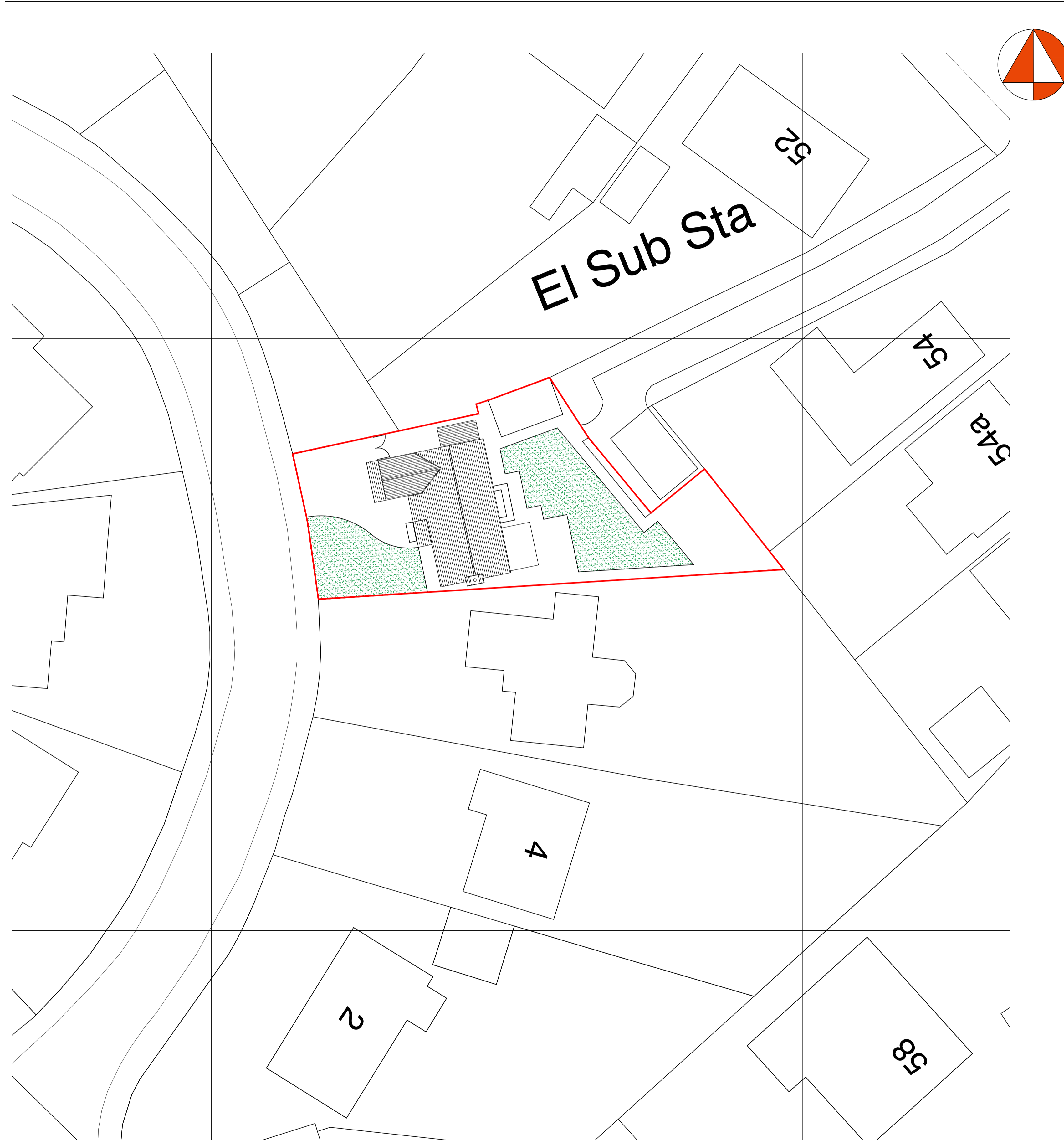
Site Plan (1:200)
