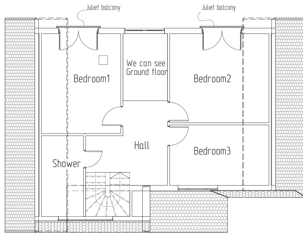
Loft Plan
