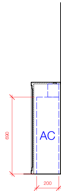
3 Section 1:20 @ A3
