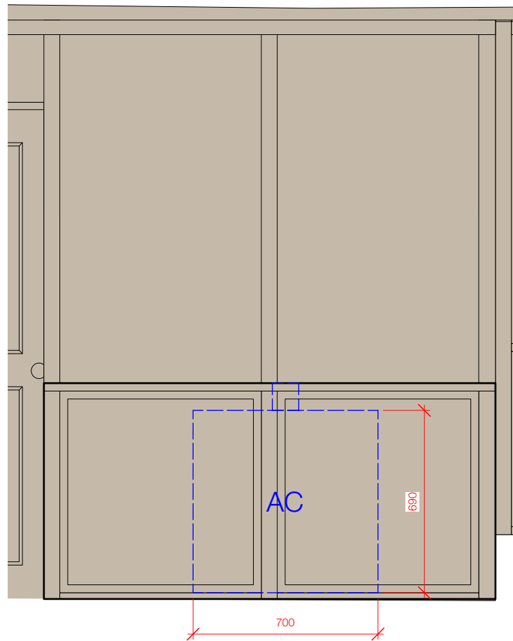
2 Elevation 1:20 @ A3
