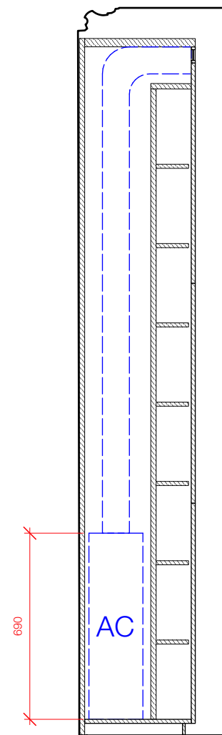
3 Section 1:20 @ A3
