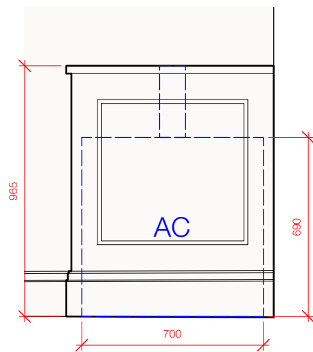
2 Elevation 1:20 @ A3
