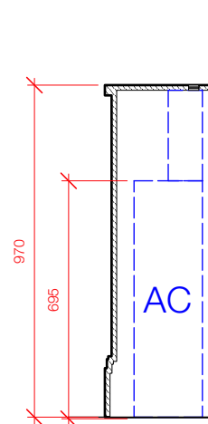
3 Section 1:20 @ A3
