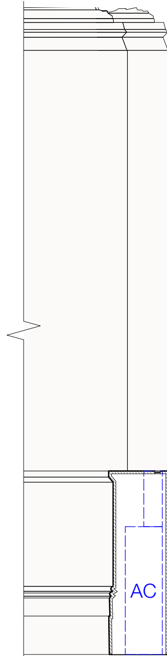
3 Section 1:20 @ A3
