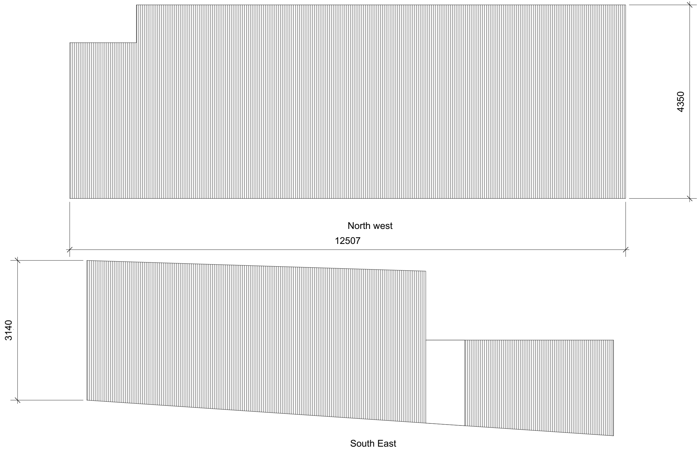
6 Existing Sides Scale: 1:50
