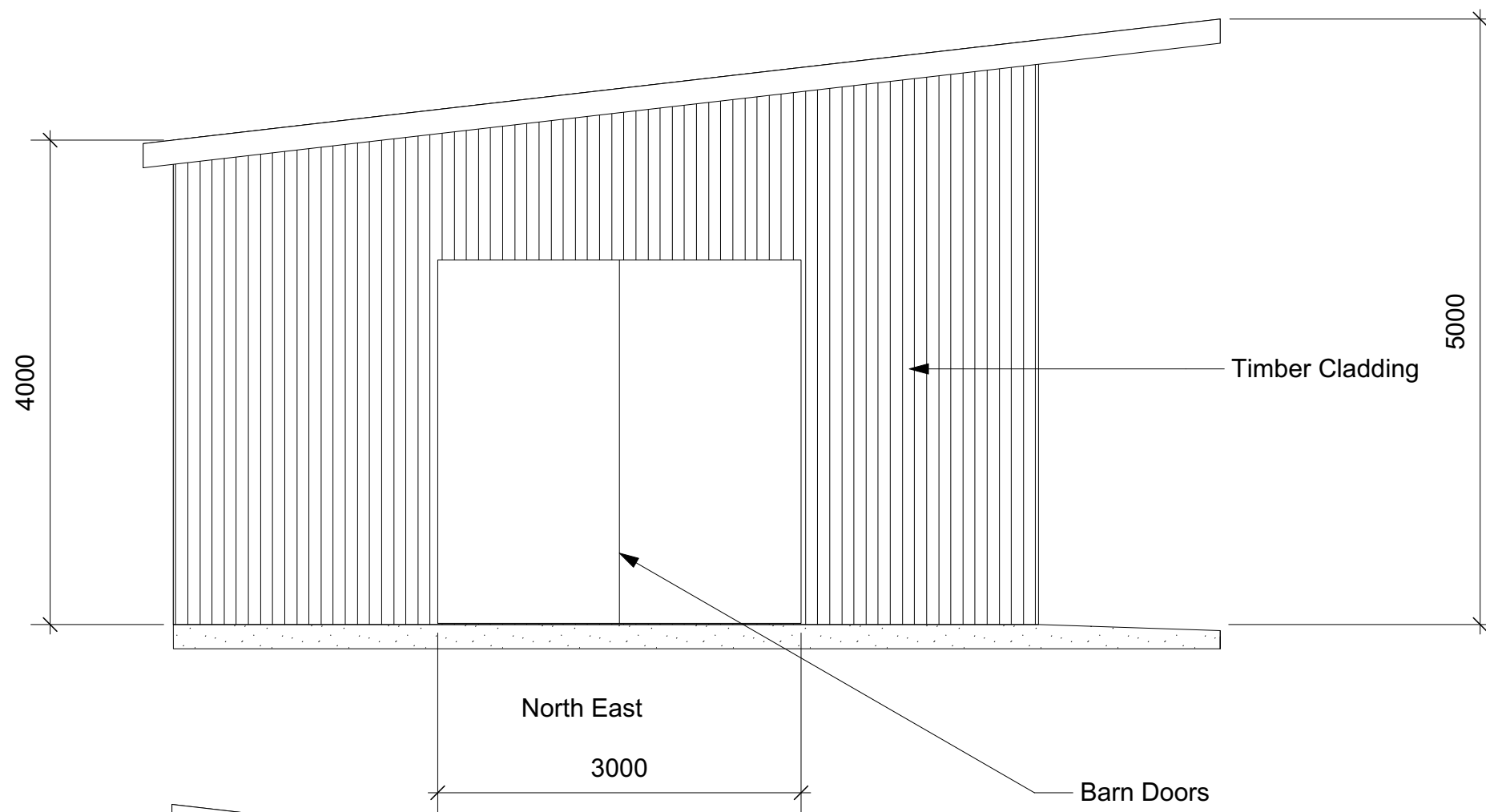
2 Elevations 2 Scale: 1:50
