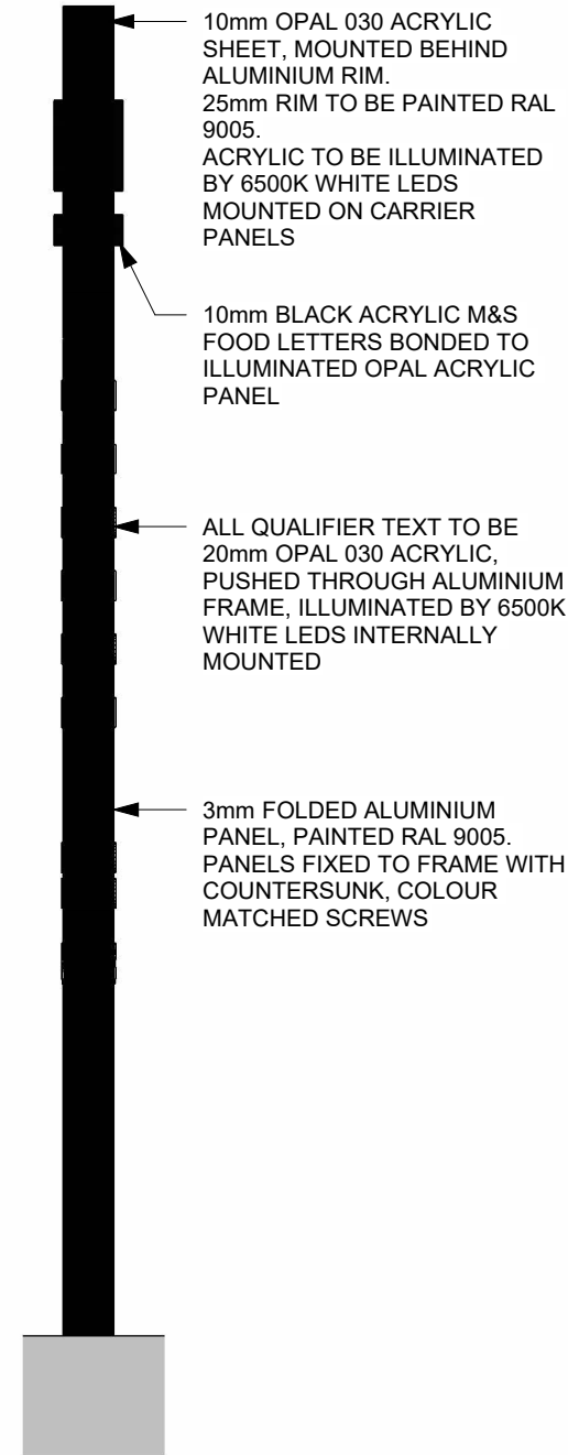
4 Totem Elevation 4 1 : 50
