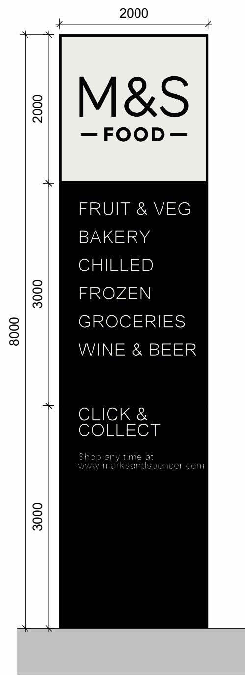
1 Totem Elevation 1 1 : 50
