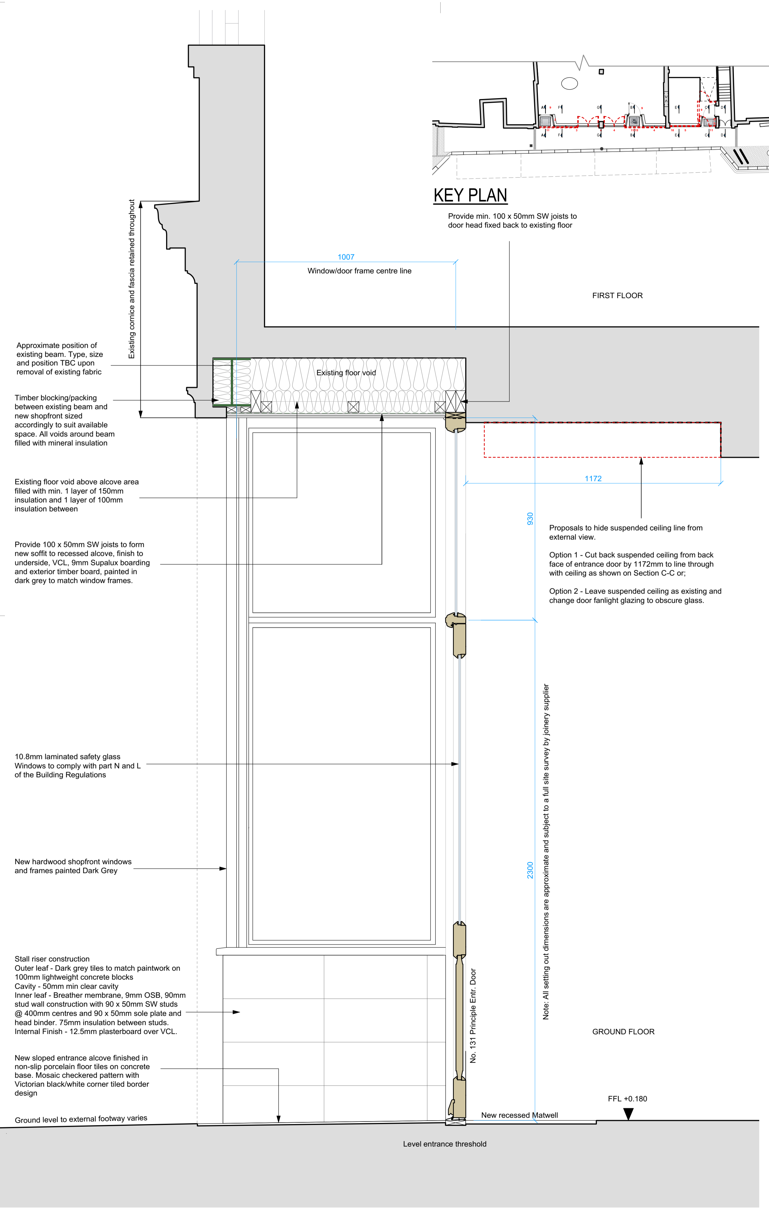
SECTION B-B 1:10 @ A1
