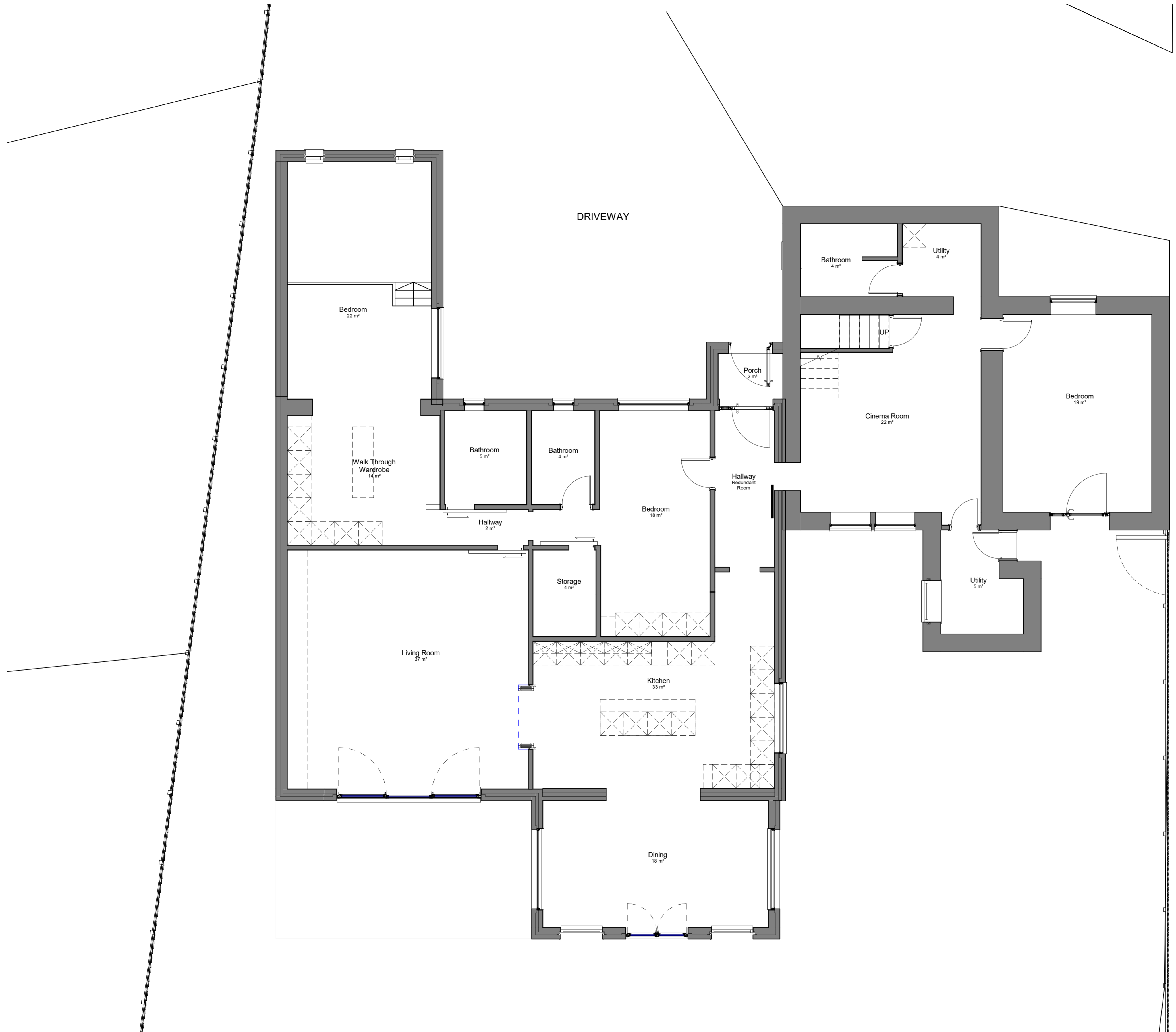
00_GROUND FLOOR 1 : 50
